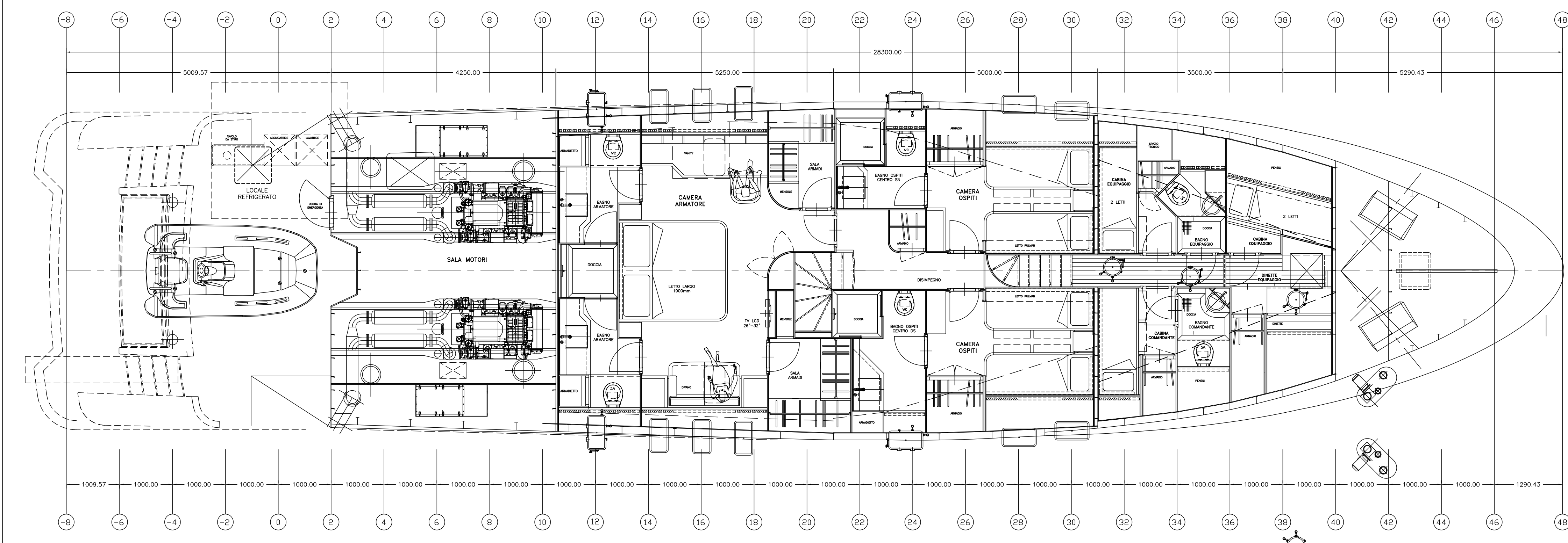
A PIANO GENERALE PIANTA PONTE SOTTOCOPERTA EQUIPAGGIO ALTERNATIVA 2
