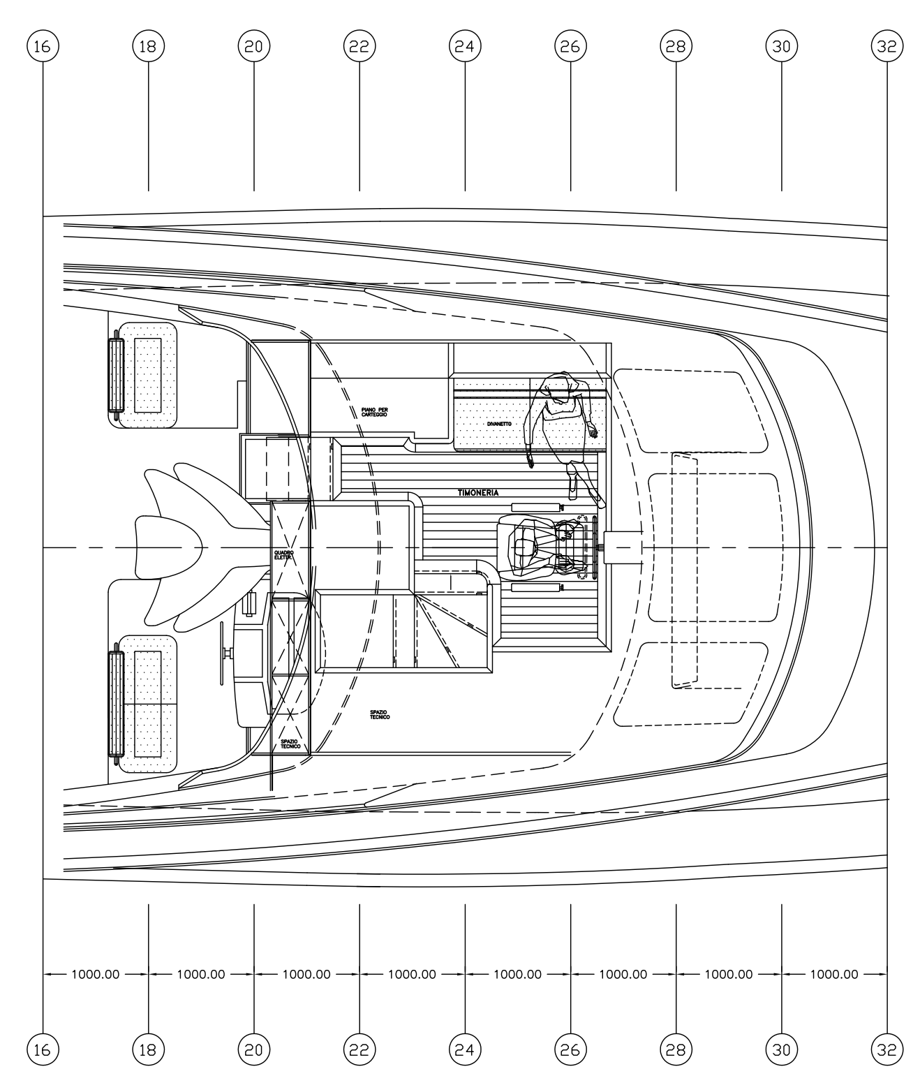
B PIANO GENERALE PIANTA TIMONERIA
