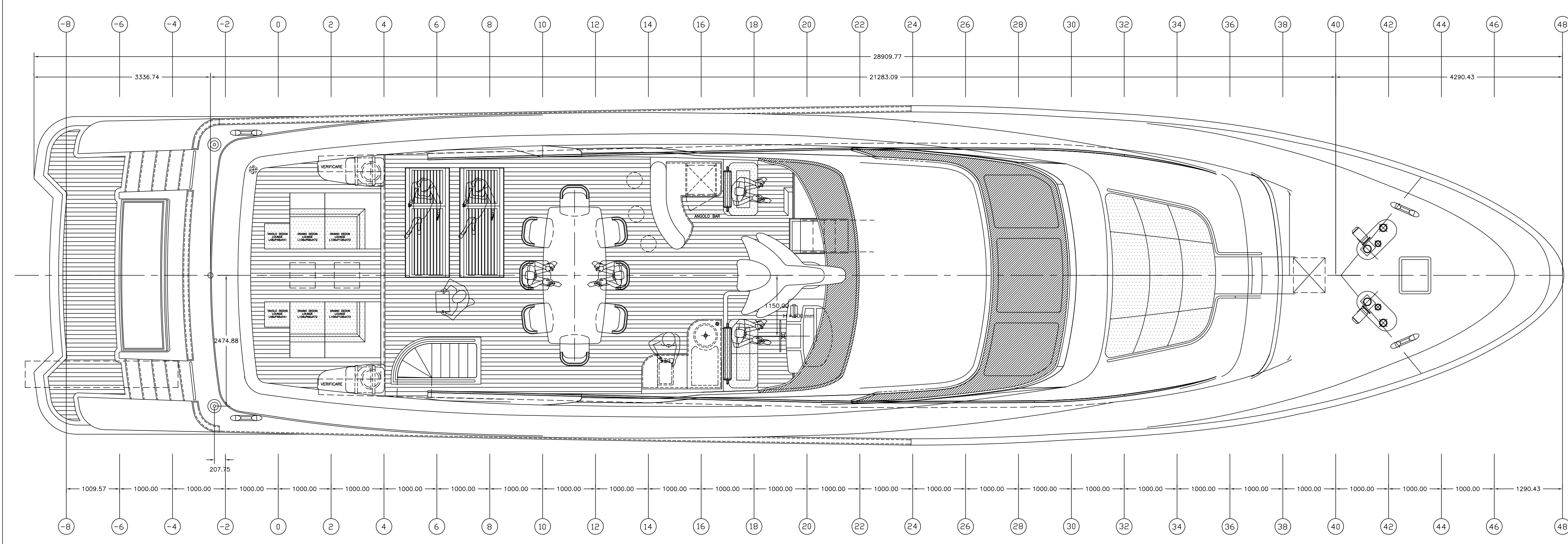
C PIANO GENERALE PIANTA PONTE FLY SALONE ALTERNATIVA 1
