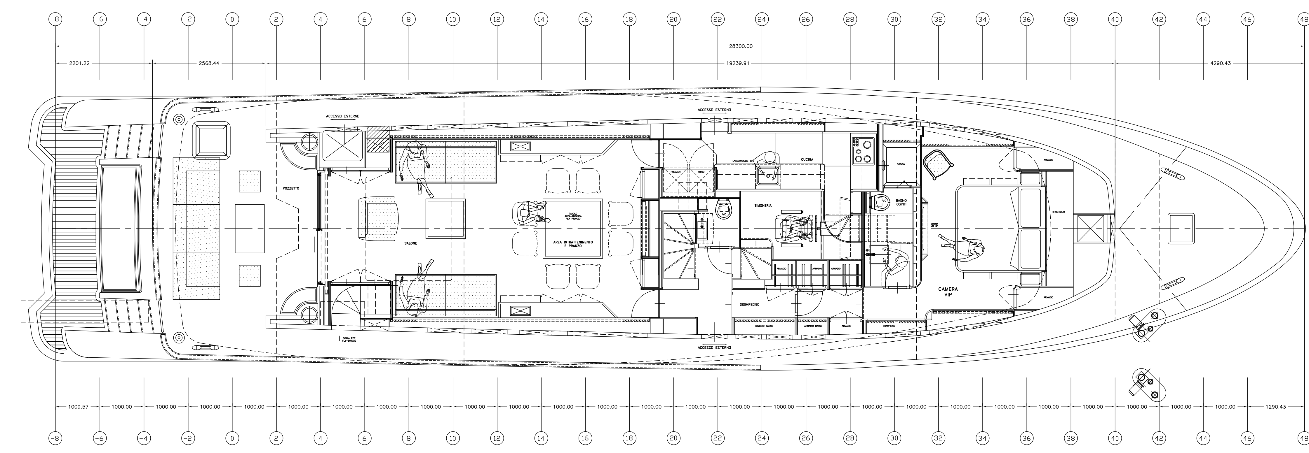
B PIANO GENERALE PIANTA PONTE COPERTA SALONE ALTERNATIVA 3
